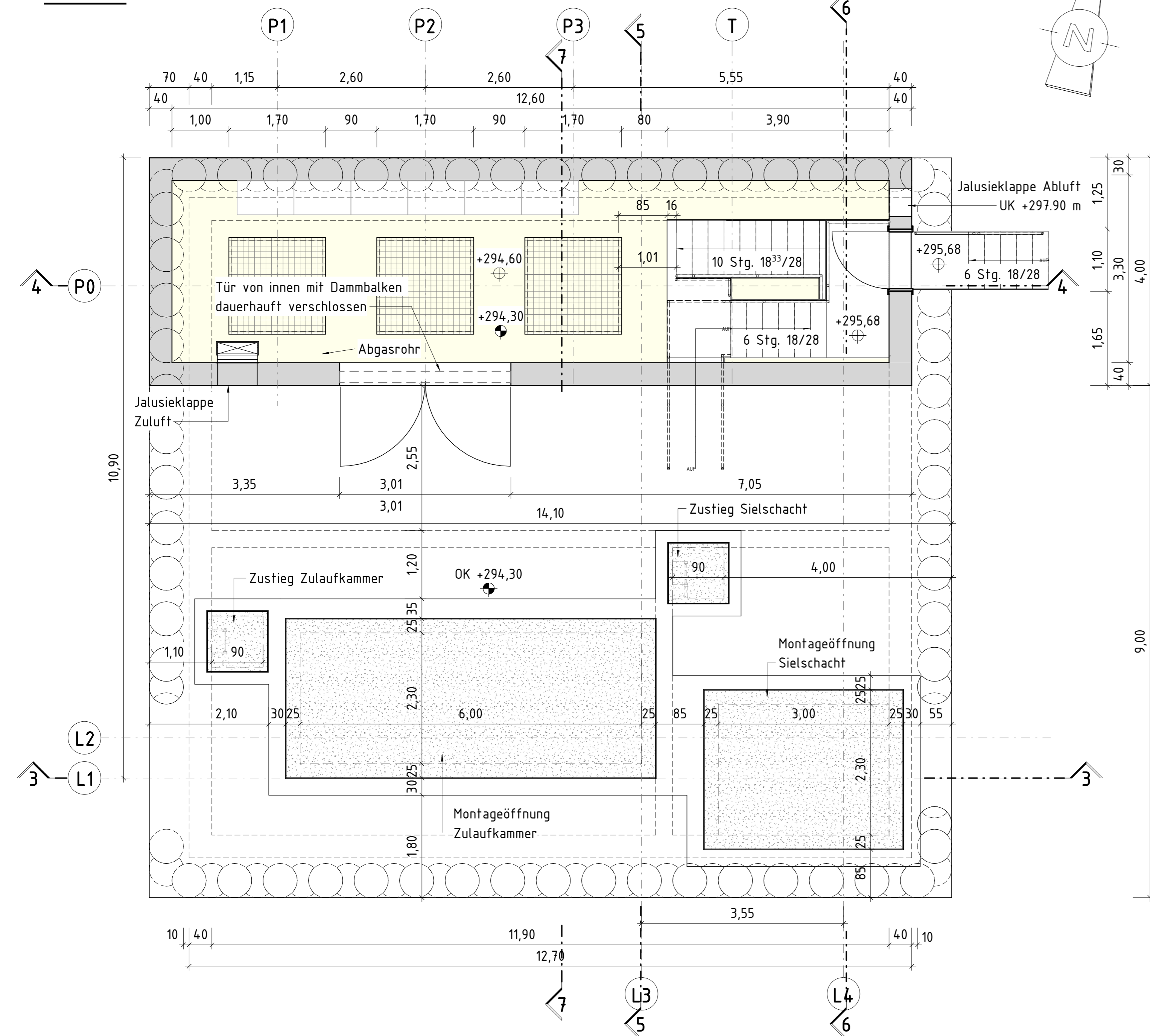
PW- GOK M. 1 : 50
