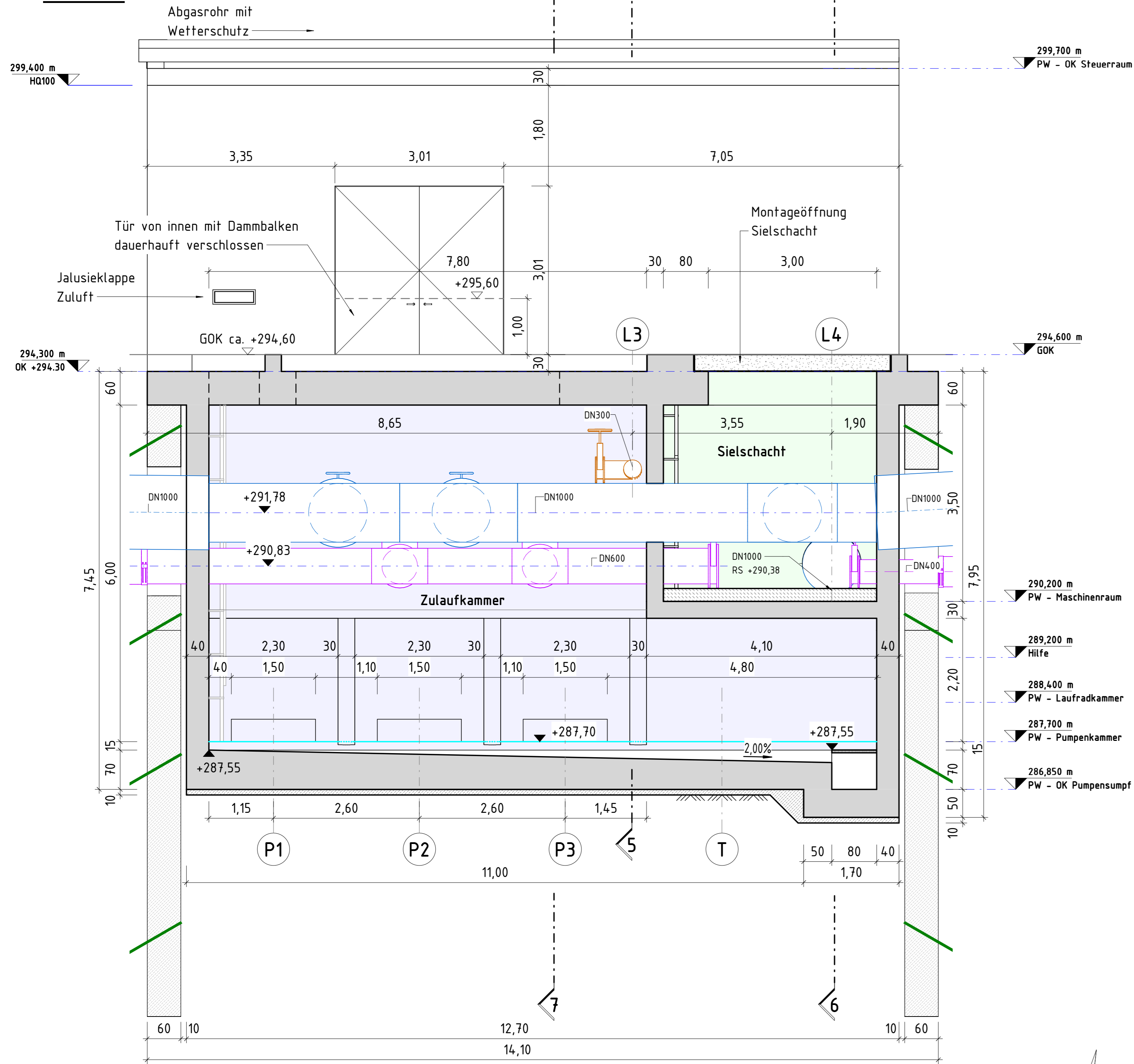
PW- GOK M. 1 : 50
