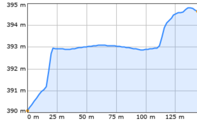
Höhenschnitt 4 (nördlicher Querschnitt des Platzes)
