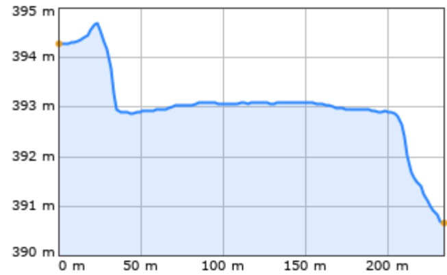
Höhenschnitt 2 (Längsschnitt des Platzes)
