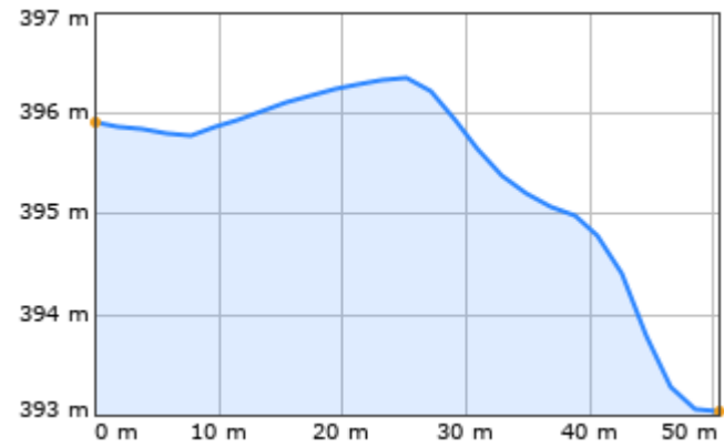
Höhenschnitt 1 (Zufahrt)
